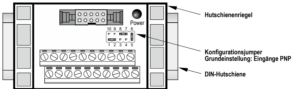
Eingänge PNP
