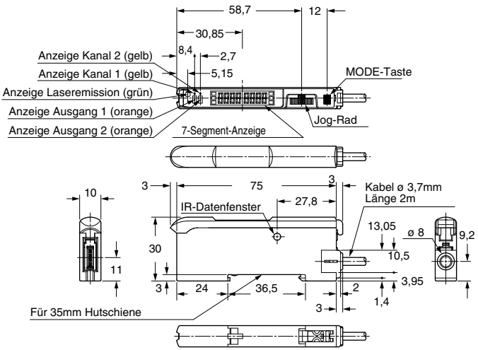
LS-401-C2 / LS-401P-C2 Steuereinheit
