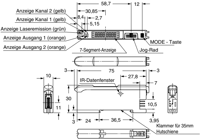
LS-401 / LS-401P Steuereinheit
