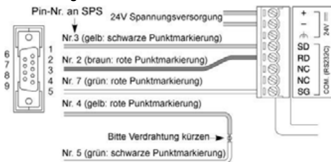
Pinbelegung SPS
