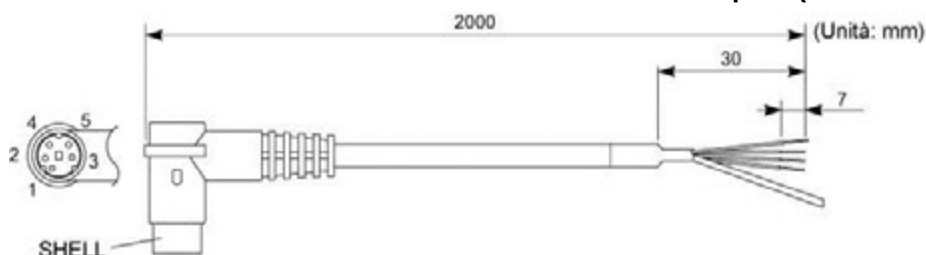
Segnale lato mini connettore DIN
